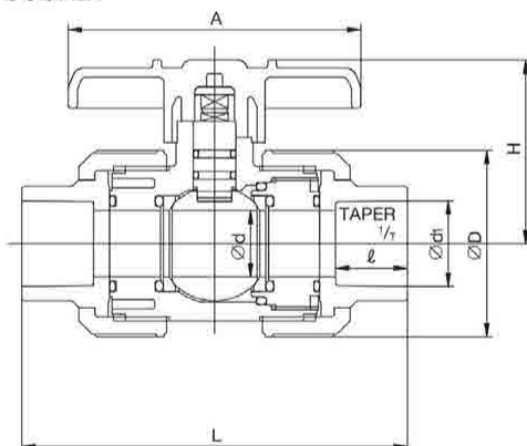
SOCKET
