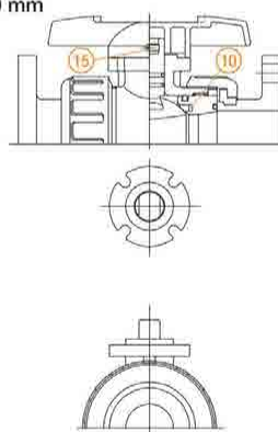
SOCKET
